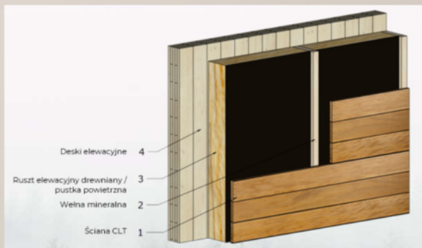
struktura ściany zewnętrznej
